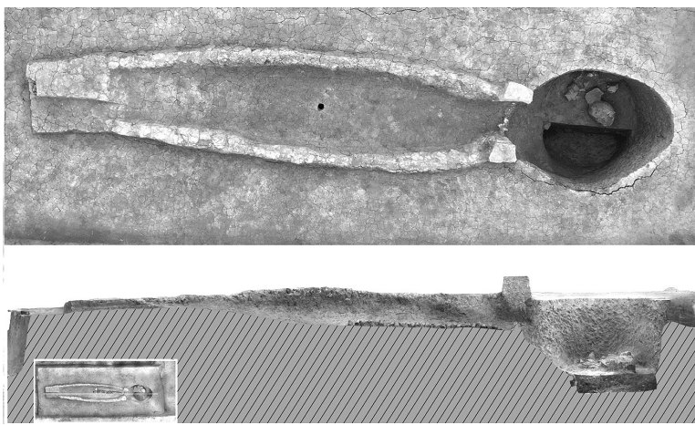
浙江舟山姚家湾一号盐灶(Y21)平剖面图(距今4000年)。
